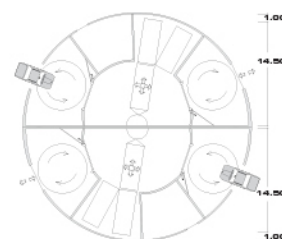
Ein- / Ausfahrtebene entry / exit level
