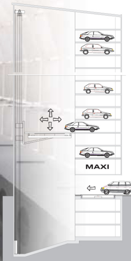
Schnitt / cross section
