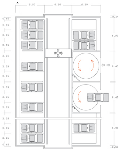
Ein- / Ausfahrtebene in / out level
