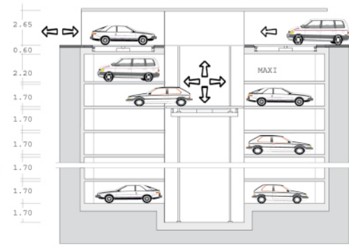
Schnitt cross section
