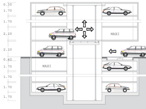
Schnitt cross section
